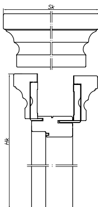
Sk – szerokość po zewnętrznej stronie korony Hk – wysokość po zewnętrznej stronie korony
